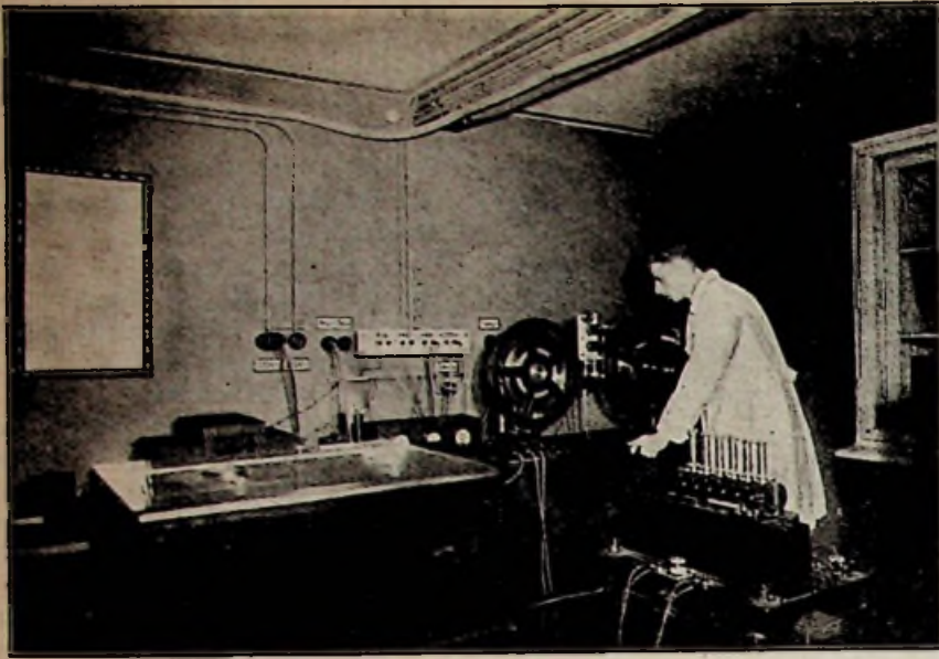
Küchenmeister-Stille installatie voor het vastleggen van het geluid op een stalen band. Men ziet duidelijk de twee „staalbandrollen”. Daar tusschen, op het witte bordje, de twee magneten. Langs de zoldering de „stofzuigerbuis” voor de gramtoonopnamen.
