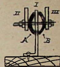
Fig. 6. A en B = 2 cuprox cellen tegen elkaar ingeschakeld. I omgebogen plaatje koper. II en III plaatje koper via een kartonnen ring vastgedrukt door het boutje met moer.
