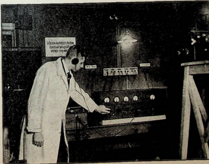
De versterker voor gramfoonopnamen. In het midden de 50 Watt versterker. Rechts de installatie voor het opnemen van gramfoonplaten in was.
